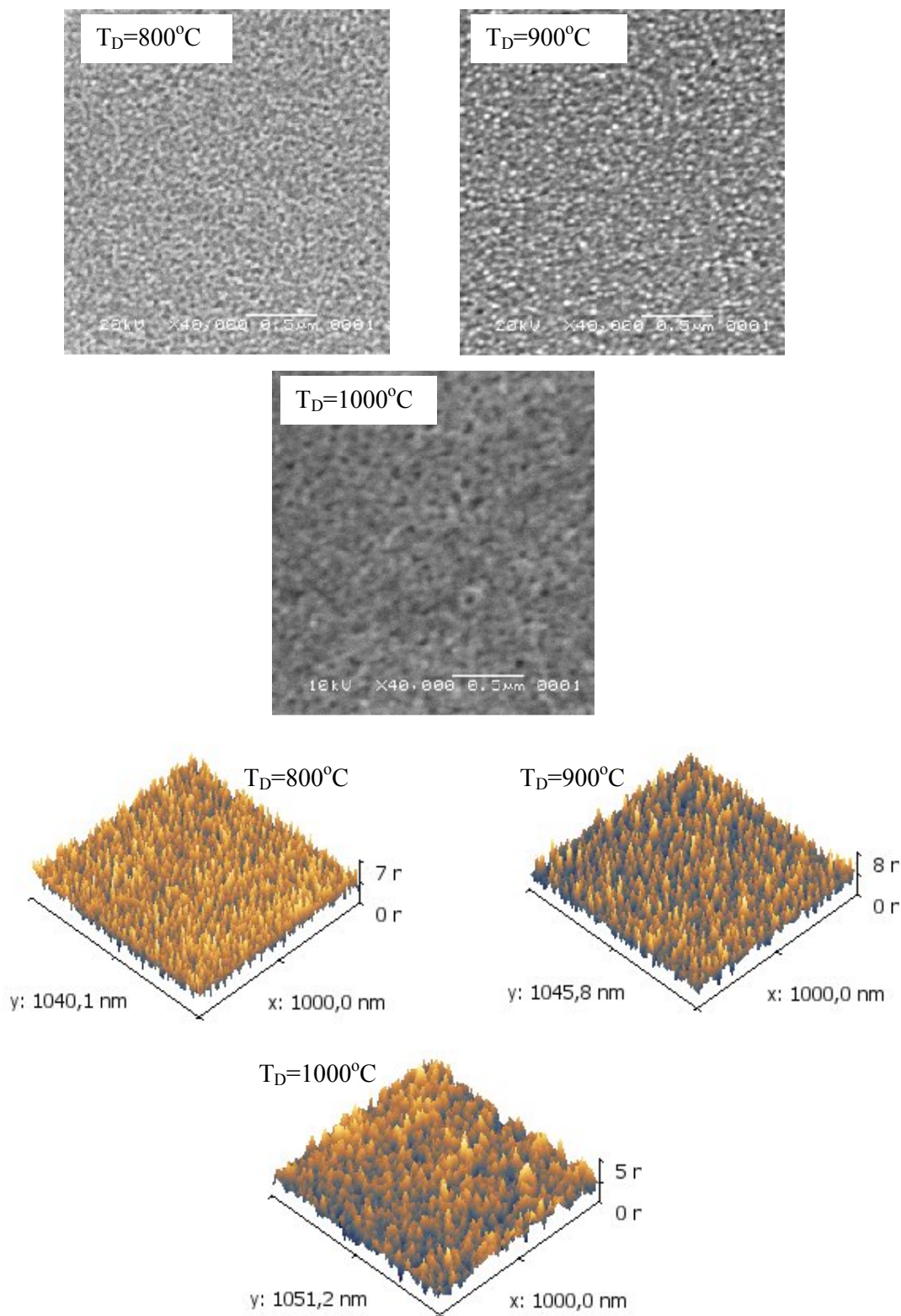
Gambar.2. Citra SEM morfologi dari film tipis GaN yang ditumbuhkan dengan variasi temperatur dekomposisi N 2 : a. 800°C b. 900°C c. 1000°C
