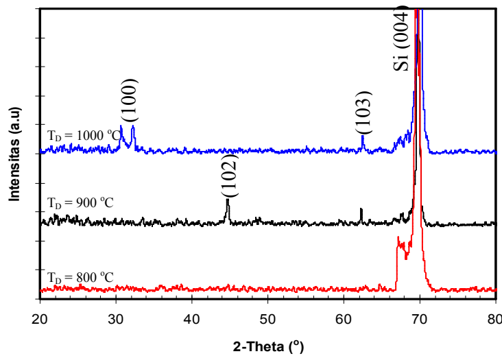
Gambar 1. Pola XRD pada lapisan tipis semikonduktor GaN yang dideposisi di atas substrat Silikon (004) pada berbagai temperatur; 800°C; 900°C; dan 1000°C
