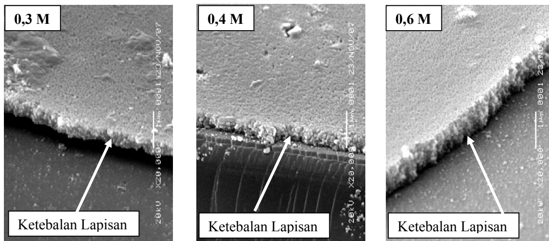
Gambar.3. Citra SEM penampang dengan perbesaran 20.000x dari film tipis GaN yang ditumbuhkan dengan variasi molaritas larutan gel kristal Ga.
