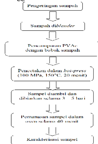
Gambar 1. Diagram alir sintesis komposit PVAc-sampah
