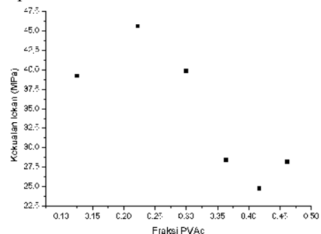
Gambar 3. Grafik kekuatan tekan terhadap fraksi sampah.
