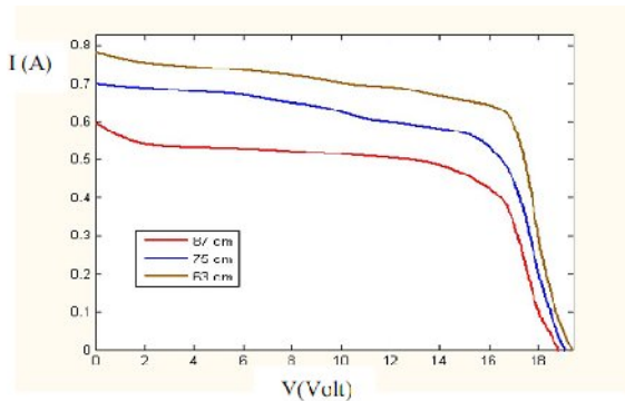
Gambar 2. kurva karakteristik I-V dengan intensitas 256,26 watt/m 2 ; 325,24 watt/m 2 dan 669,3 watt/m 2 pada jarak 87 cm dalam ruang kaca.
