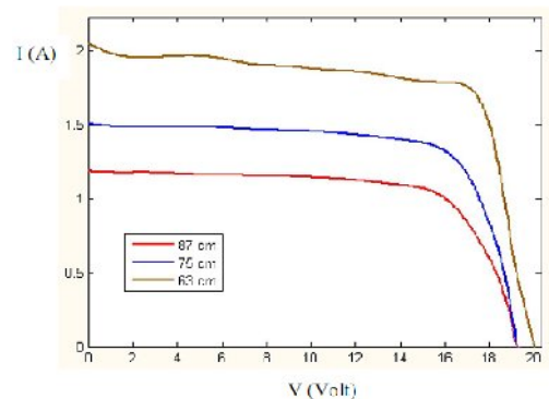
Gambar 4. kurva karakteristik I-V tanpa ruang cermin.
