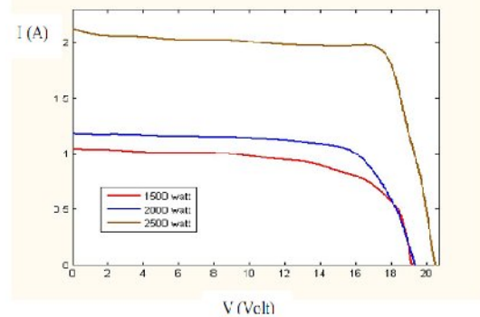
Gambar 3. kurva karakteristik I-V pada ruang cermin
