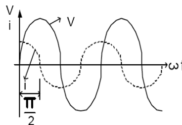
Gambar 11. Hubungan Fasa Antara Arus Dan Tegangan Pada Beban Kapasitif
