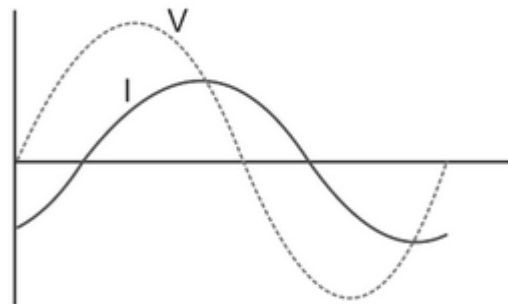
Gambar 9. Beban Induktif
