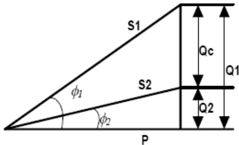
Gambar 11. Prinsip Perbaikan Faktor Daya
