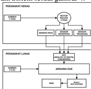
Gambar 4. Diagram blok sistem
