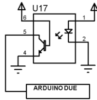
Gambar 7. Rangkaian Sensor optocoupler
