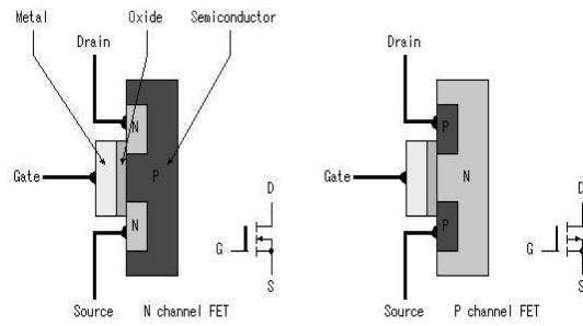
Gambar 3 Prinsip kerja MOSFET tipe NPN
