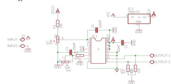
Gambar 7. Rangkaian Kontrol
