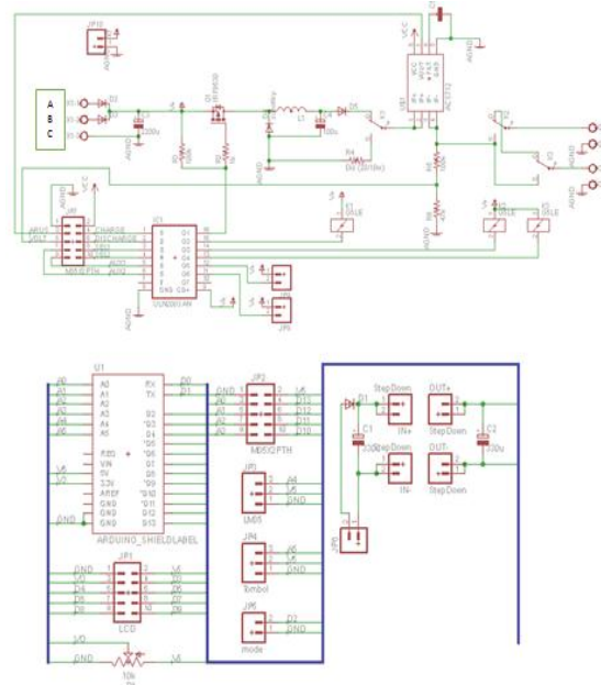
Gambar 4. Rangkaian Keseluruhan
