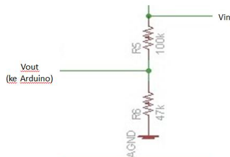
Gambar 1 Rangkaian pembagi tegangan
