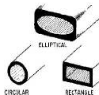
Gambar 1. Jenis Waveguide
