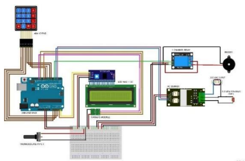
Gambar 2. Rangkaian Keseluruhan Sistem
