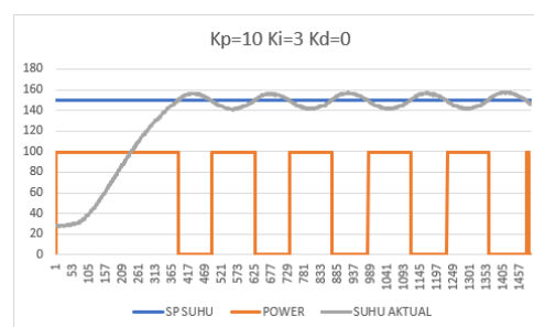
Gambar 5. Grafik Sistem Dengan Nilai Kp Lebih Besar
