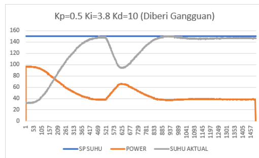
Gambar 8. Grafik Hasil Pengujian Sistem Dengan Kontrol PID Pada Suhu 150^{\circ}\text{C} dengan gangguan
