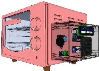
Gambar 2. Rangkaian Keseluruhan Sistem
