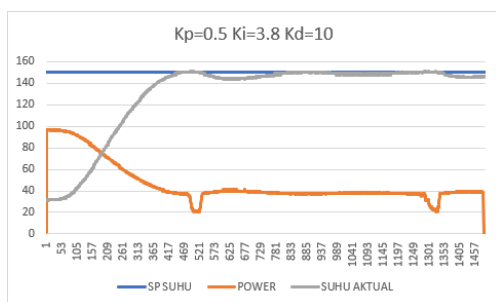
Gambar 7. Grafik Hasil Pengujian Sistem Dengan Kontrol PID Pada Suhu 150^{\circ}\text{C}
