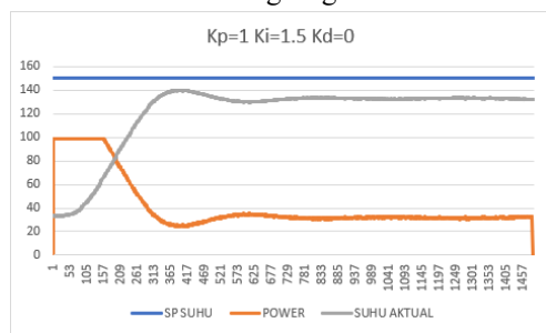
Gambar 6. Grafik Sistem Dengan Nilai K_p Lebih Kecil
