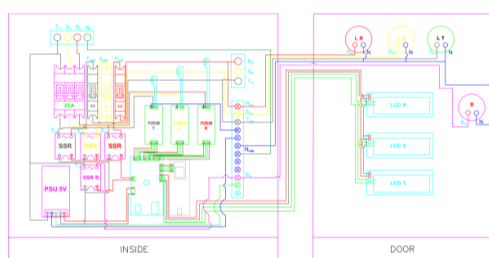
Gambar 2. Rangkaian Keseluruhan Sistem
