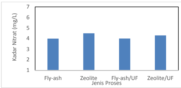
Gambar 4. Kadar nitrat dalam filtrat hasil proses menggunakan adsorben dan kombinasinya dengan ultrafiltrasi
