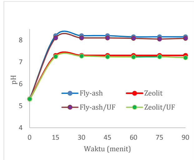
Gambar 2 Pengaruh waktu terhadap pH filtrat pada laju alir umpan UF sebesar 4L/menit
