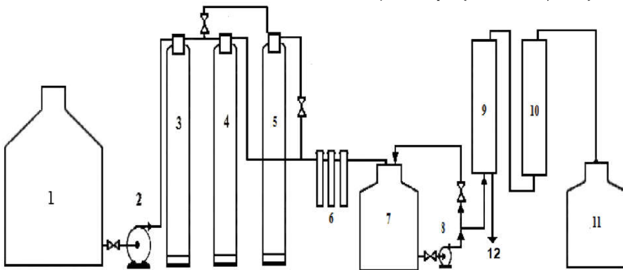
Gambar 1 Skema peralatan
