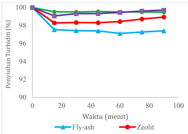
Gambar 3 Pengaruh waktu terhadap persentase penyisihan turbiditi
