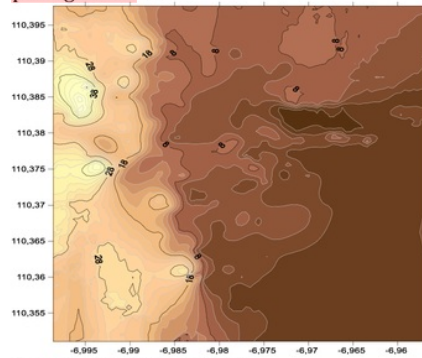
Gambar 2c : Sebaran fosfat
