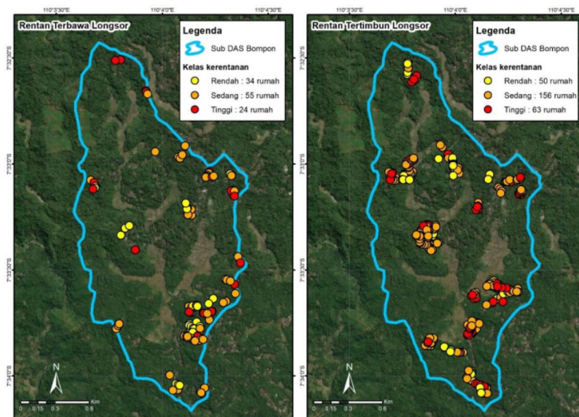
Gambar 7. Peta kerentanan fisik rumah terhadap longsor dalam skala rumah tangga di Sub-DAS Bompon
