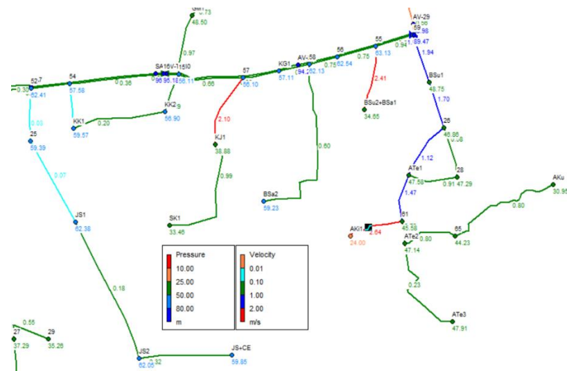
Gambar 11. Hasil simulasi kecepatan alternatif satu
