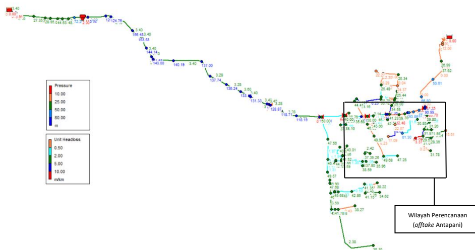
Gambar 5. Hasil simulasi Jaringan Distribusi Utama (JDU) eksisting IPA Cikalong sampai offtake Antapani
