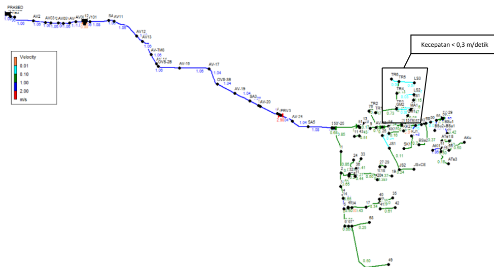
Gambar 8. Hasil simulasi kecepatan
