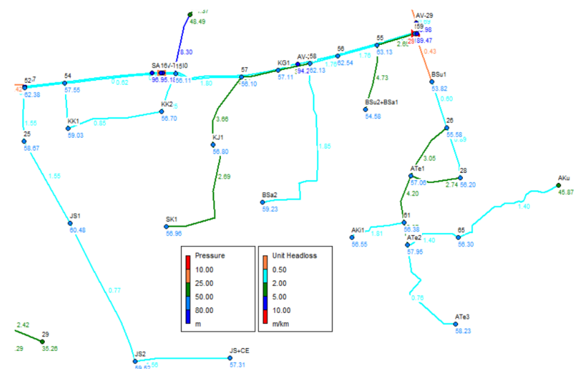
Gambar 15. Hasil simulasi headloss alternatif dua
