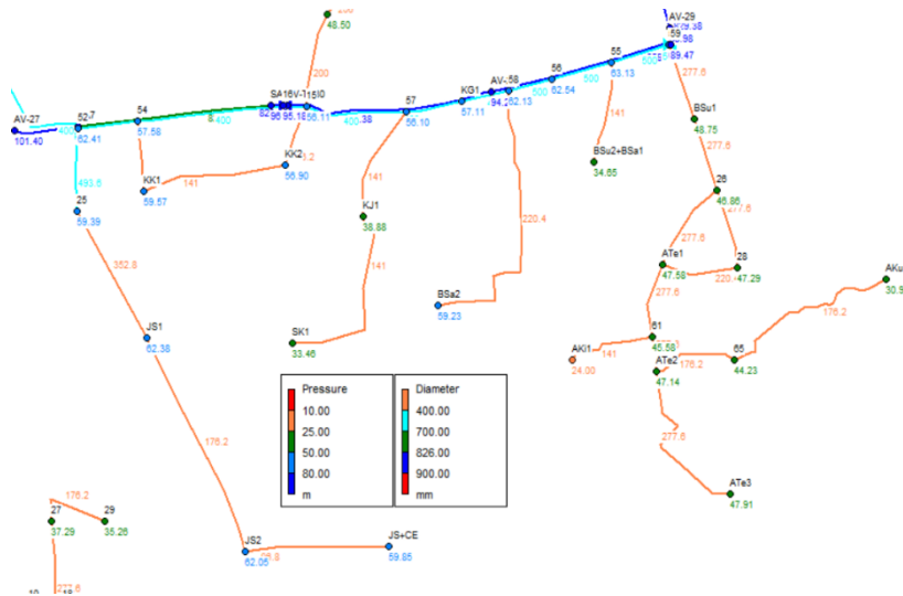
Gambar 10. Hasil simulasi sisa tekan alternatif satu
