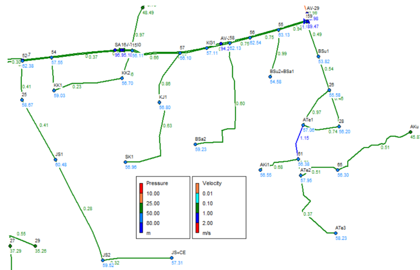
Gambar 14. Hasil simulasi kecepatan alternatif dua
