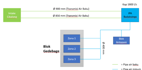
Gambar 2. Skema jaringan distribusi awal
