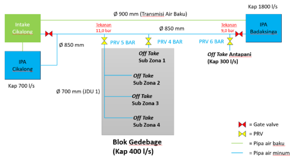
Gambar 6. Skema jaringan distribusi utama dari IPA Cikalong offtake Antapani
