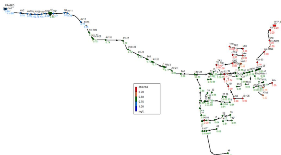
Gambar 16. Hasil simulasi konsentrasi sisa khlor jaringan distribusi utama (JDU)
