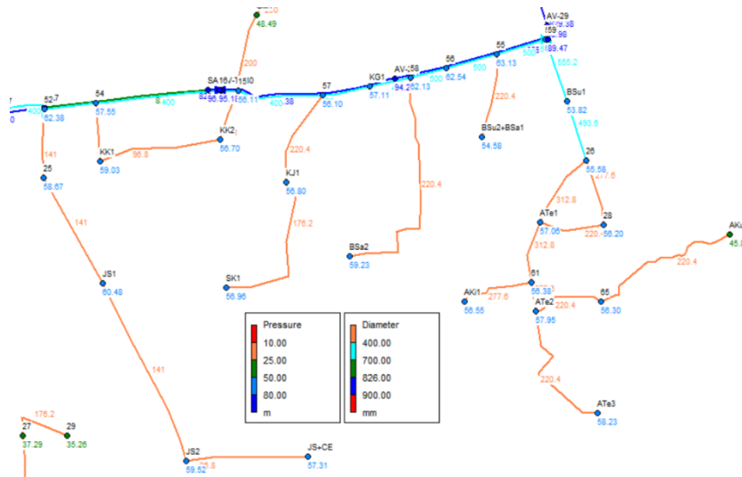
Gambar 13. Hasil simulasi sisa tekan alternatif dua
