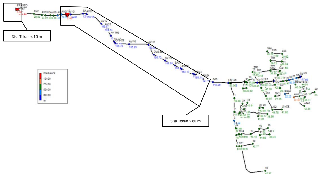
Gambar 7. Hasil simulasi sisa tekan
