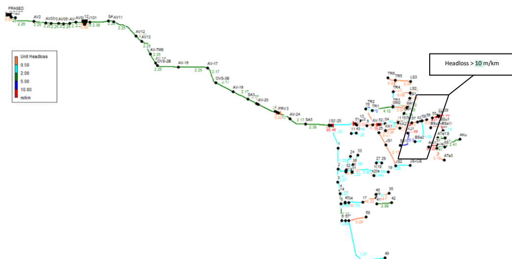
Gambar 9. Hasil simulasi hilang tekan ( headloss )
