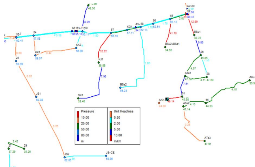
Gambar 12. Hasil simulasi headloss alternatif satu
