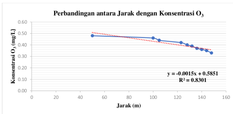
Gambar 5. Perbandingan pengaruh Jarak dan Konsentrasi O_3 .
