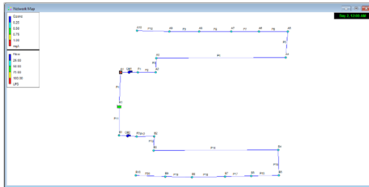
Gambar 4. Hasil Simulasi Hidrolis dan Konsentrasi Ozone pada Jam ke-24 Sumber. hasil elaborasi penulis (2021).
