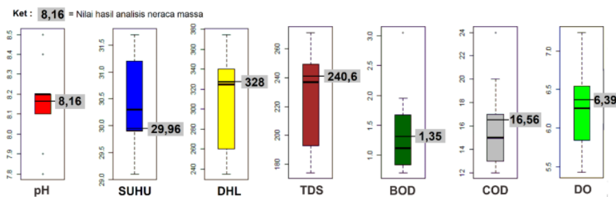
Gambar 2. Diagram Boxplot setiap parameter kualitas air beserta hasil nilai analisis neraca massa. Tingginya nilai BOD dan COD di Lokasi 2 karena adanya tambahan bahan pencemar hasil limbah pabrik triplek yang masuk dalam sistem aliran Sungai Arjasa. Semakin ke arah hilir dari
