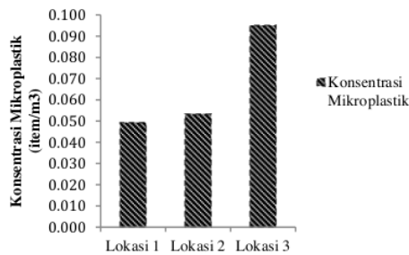
Gambar 2. Konsentrasi Mikroplastik
