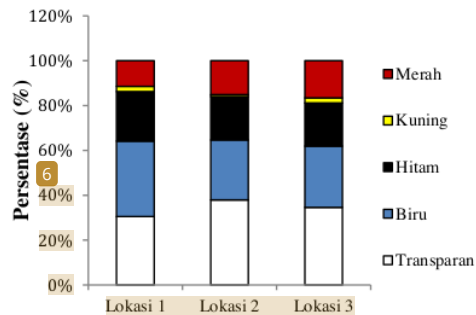
Gambar 5. Warna Mikroplastik
