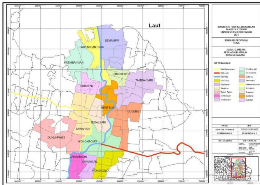
Gambar 1. Lokasi Penelitian
