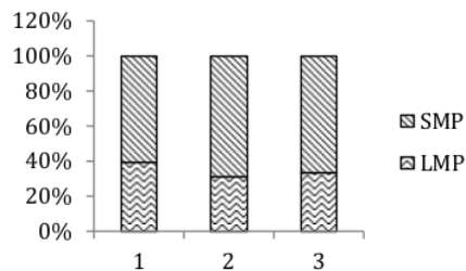
Gambar 7. Ukuran Mikroplastik
