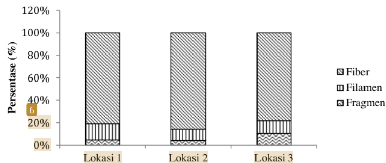
Gambar 3. Bentuk Mikroplastik
