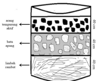
Gambar 1. Penampang Media Filtrasi
