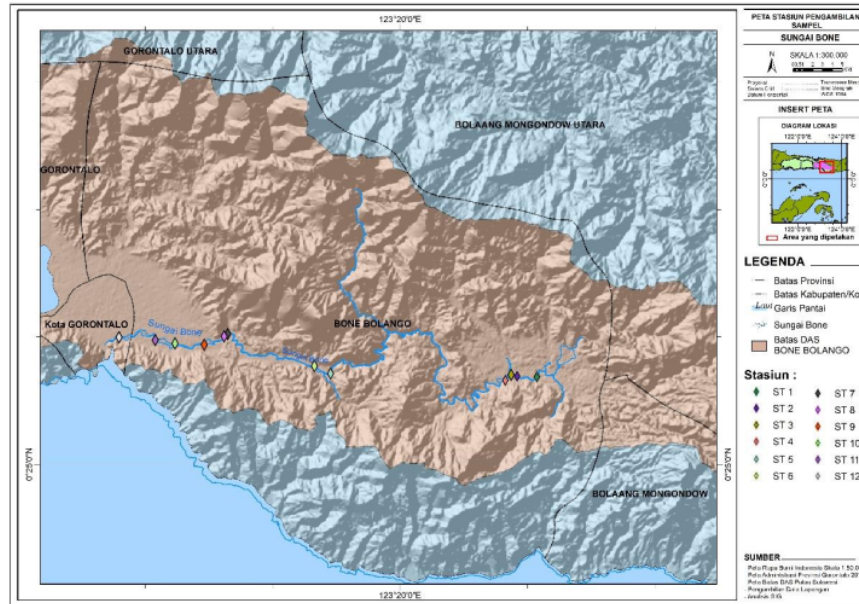
Gambar 1. Peta lokasi penelitian yang menunjukkan 12 stasiun pengamatan di Sungai Bone
