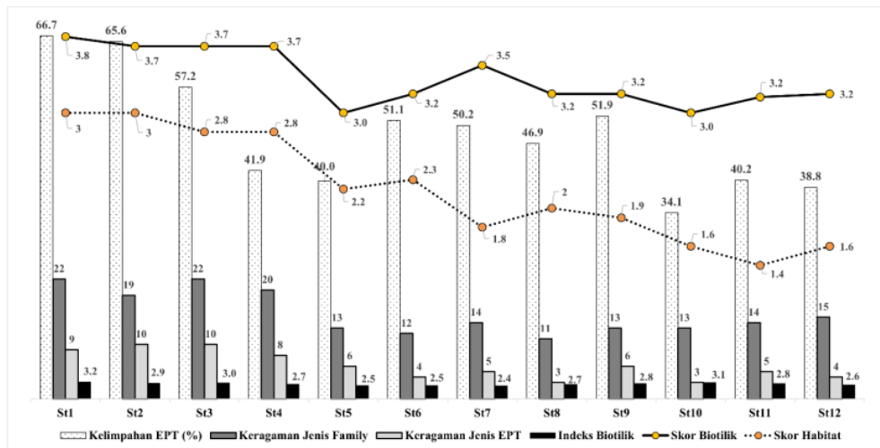
Gambar 2. Grafik Hasil pemeriksaan kondisi habitat fisik dan kualitas perairan Sungai Bone dimana kategori kondisi habitat fisik berdasarkan skor: sehat (2,4-3,0); kurang sehat (1,7-2,3); tidak sehat (1,0-1,6) sedangkan kategori pencemaran kualitas perairan berdasarkan skor biotilik: tidak tercemar (3,3-4,0); ringan (2,6-3,2); sedang (1,8-2,5); berat (1,0-1,7).
