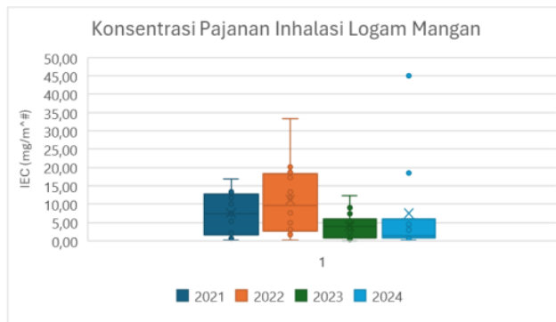
Gambar 6. Grafik hasil penilaian pajanan IEC untuk logam Mn pada pekerja pengelasan.
