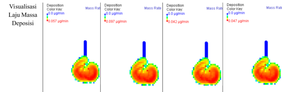
Gambar 10. Visualisasi Laju Massa Deposisi pada Tracheobronchial (TB) Saluran Pernapasan Pekerja Pengelasan untuk Total Fume
