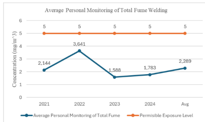
Gambar 7. Grafik Rata-rata Konsentrasi Pajanan Total Fume Pada Pekerja Pengelasan.
