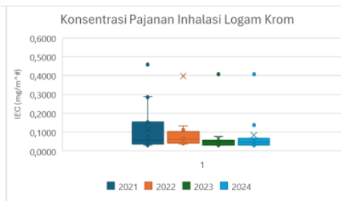
Gambar 3. Grafik hasil penilaian pajanan IEC untuk logam Cr pada pekerja pengelasan.
