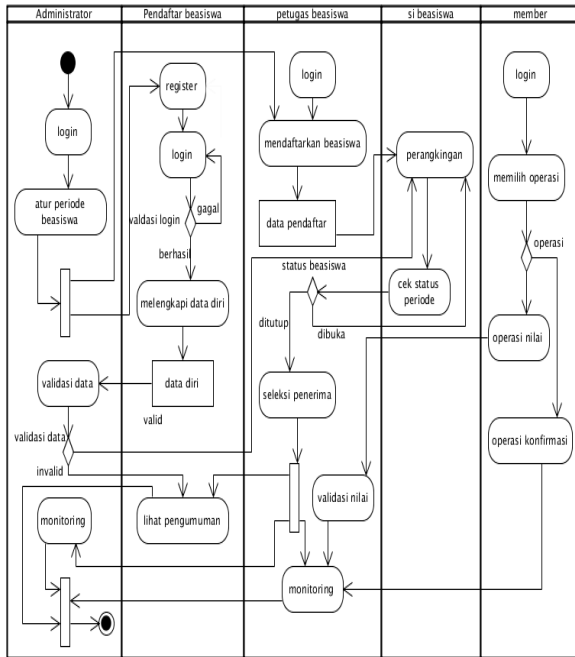
Gambar 3.1 Activity Diagram Sistem Informasi Beasiswa
