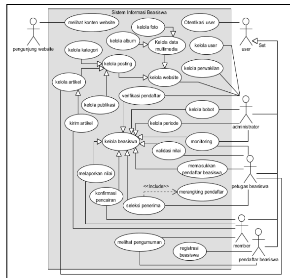
Gambar 3.4 Use Case Diagram Sistem Informasi Beasiswa Fase Elaboration
