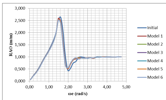
Gambar 15. RAO Gerak haluan Relatif
