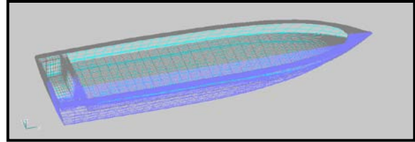
Gambar 6. Simulasi FEA
