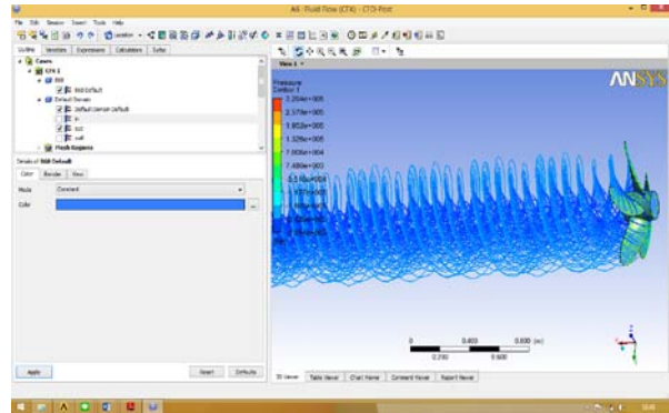
Gambar 11. Streamline velocity pada Propeller B5 50 Series (sudut rake: 10 0 Diameter: 0,813m)
