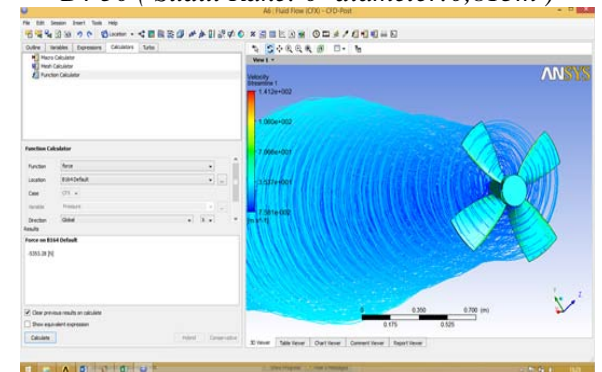
Gambar 13. Streamline velocity pada Propeller Ka4 50 Series ( Sudut Rake: 0 0 diameter: 0813m)
