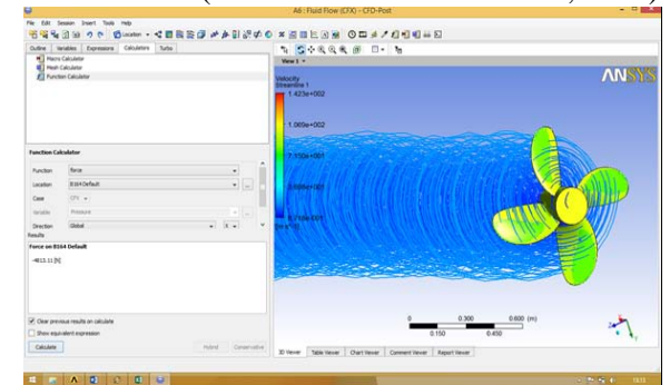
Gambar 12. Streamline velocity pada Propeller B4 50 ( Sudut Rake: 0 0 diameter:0,813m )
