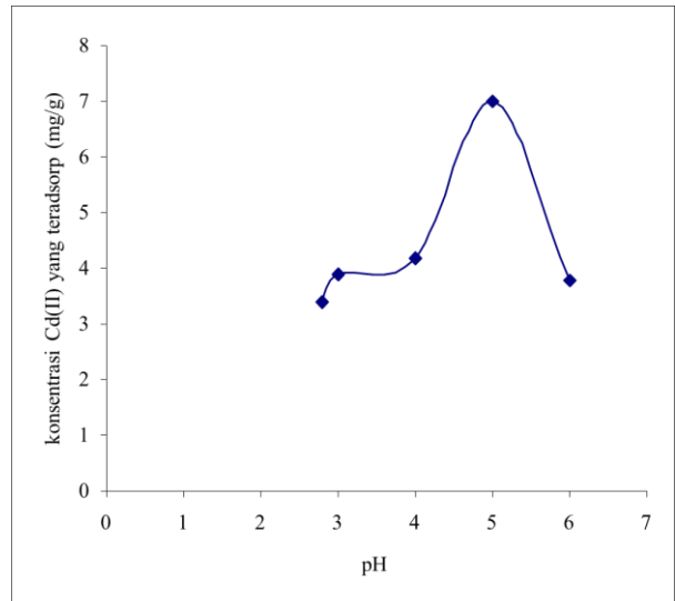
Gambar 4. Grafik Cd(II)
