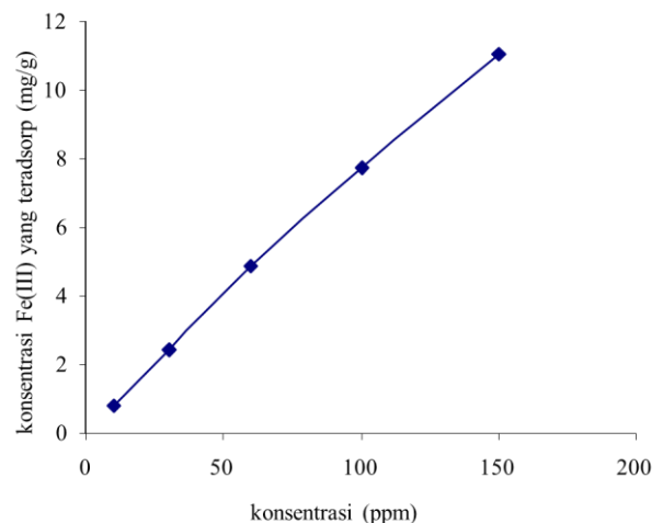
Gambar 5 Grafik adsorpsi ion Fe(III) dengan variasi konsentrasi
