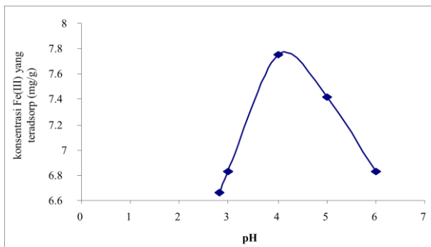
Gambar 3. Grafik Fe(III)
