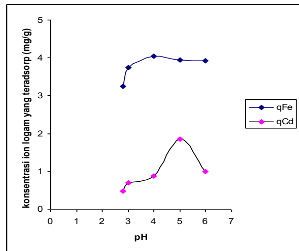
Gambar 9 Grafik uji selektifitas gel kitosan
