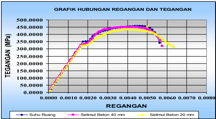
Gambar 11. Grafik hubungan Regangan -Tegangan pada elemen Balok
