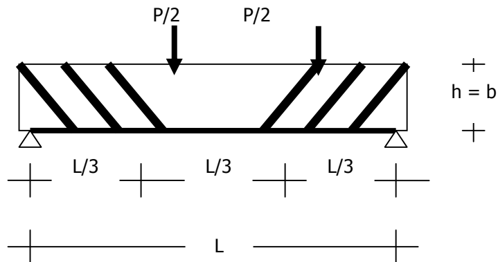
Gambar 5. Setting – up pengujian balok pasca kebakaran dengan perbaikan dengan CFS
