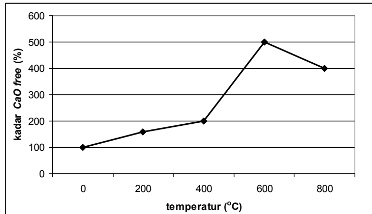
Gambar 2. Grafik hubungan antara temperatur dan kadar CaO free (Rahma, 2000)
