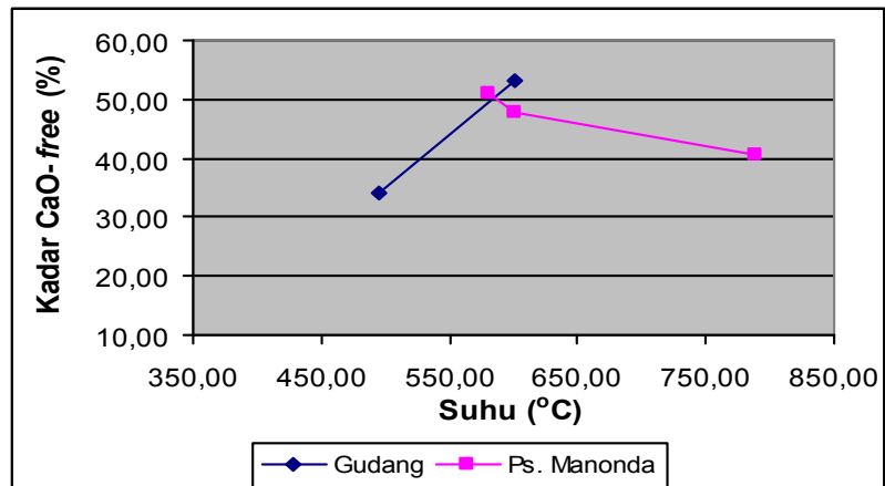
Gambar 10. Grafik hubungan antara suhu dan kadar CaO-free
