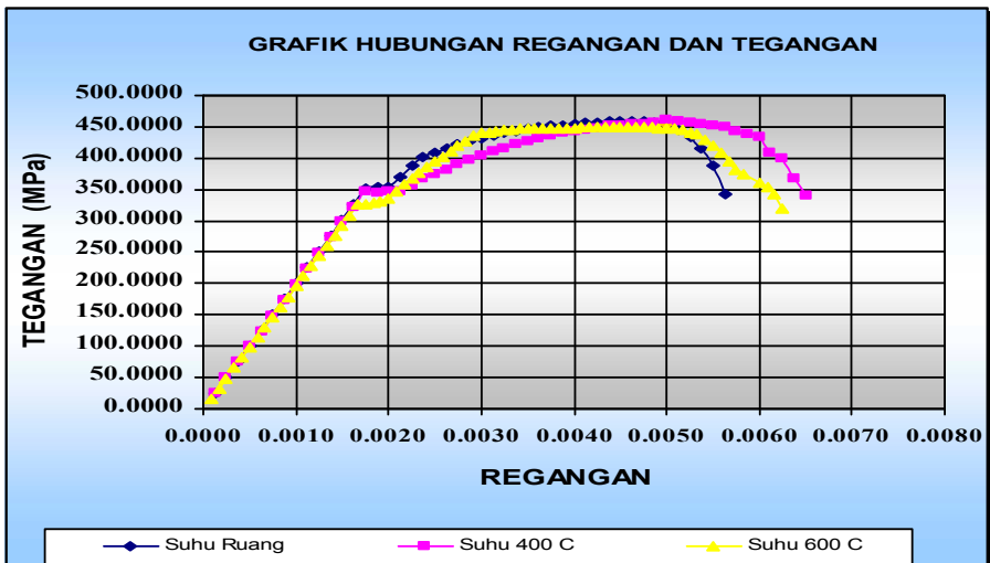
Gambar 12. Grafik hubungan Regangan - Tegangan pada elemen Kolom
