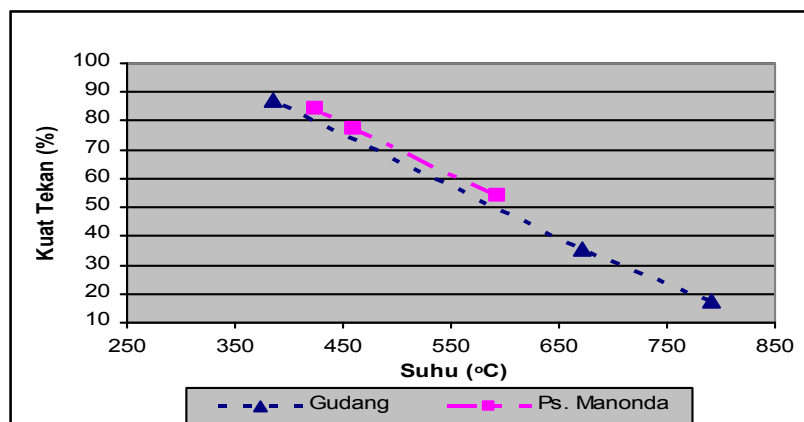
Gambar 11. Degradasi kuat tekan sampel Ruko Gudang dan Pasar Sentral Manonda
