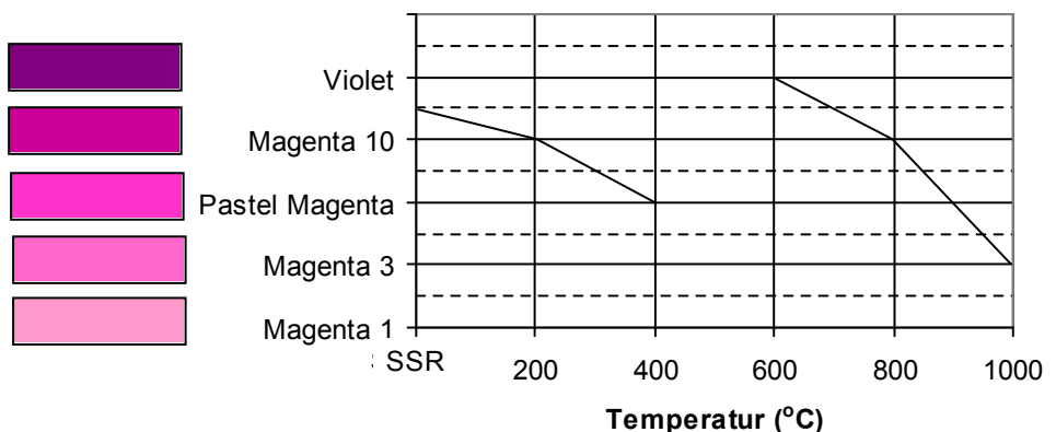
Gambar 3. Hubungan temperatur dengan indikator warna dengan Phenolphthalein
