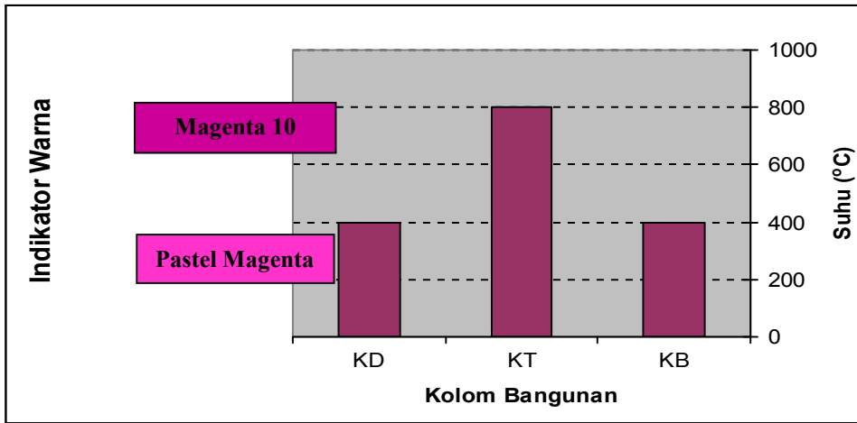
Gambar 8. Grafik hubungan perubahan warna dengan suhu kebakaran
