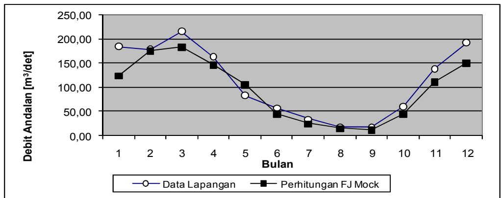
Gambar 2. Perbandingan Data Lapangan dan Perhitungan FJ Mock k=0.6
