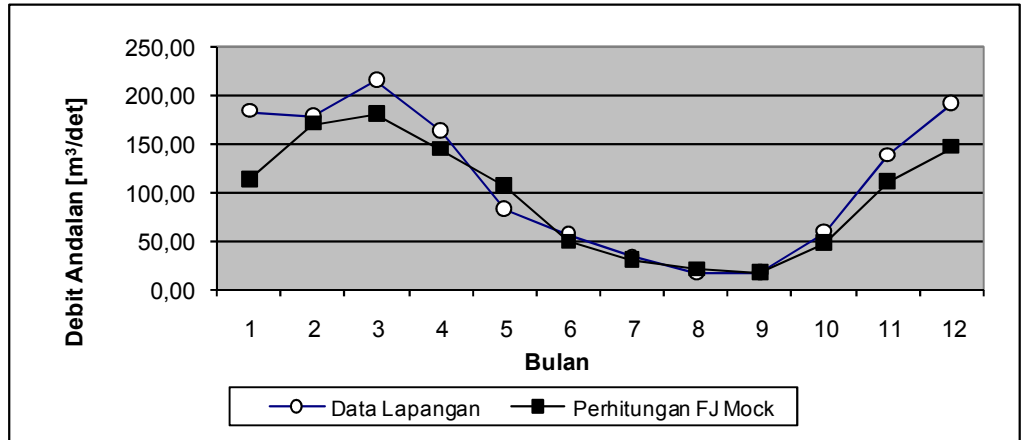
Gambar 4. Perbandingan Data Lapangan dan Perhitungan FJ Mock k=0.68
