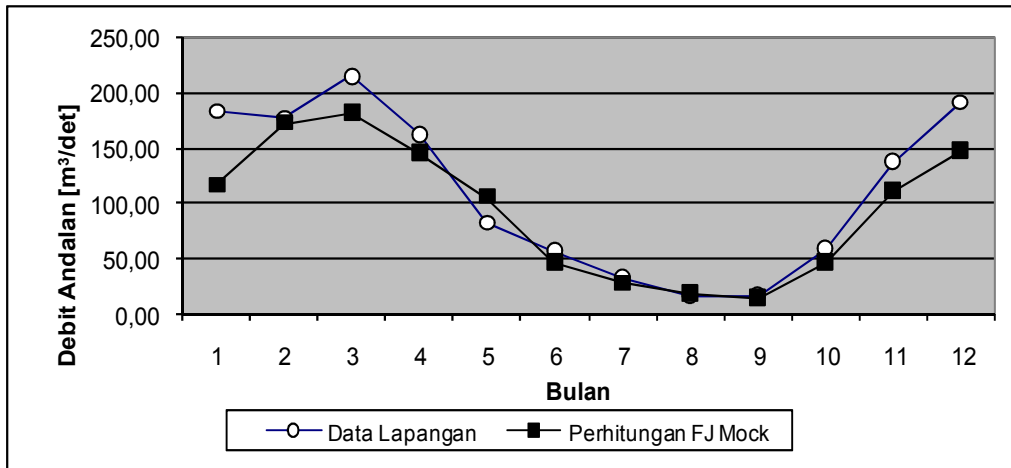
Gambar 3. Perbandingan Data Lapangan dan Perhitungan FJ Mock k=0.65
