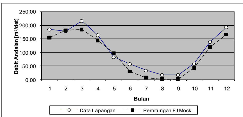
Gambar 1. Perbandingan Data Lapangan dan Perhitungan FJ Mock k=0.3
