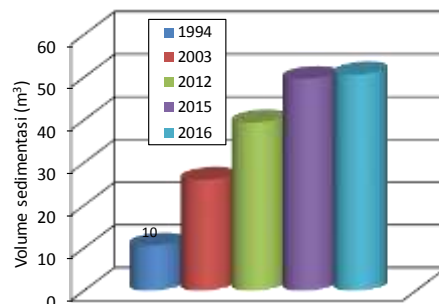
Gambar 10. Volume sedimentasi Waduk Kedungombo
