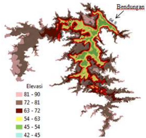
Gambar 5. DTM Waduk Kedumombo 2012
