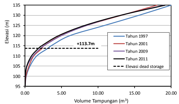
Gambar 9. Kurva karakteristik Waduk Sermo
