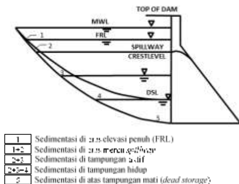
Gambar 1. Zona sedimentasi di waduk
