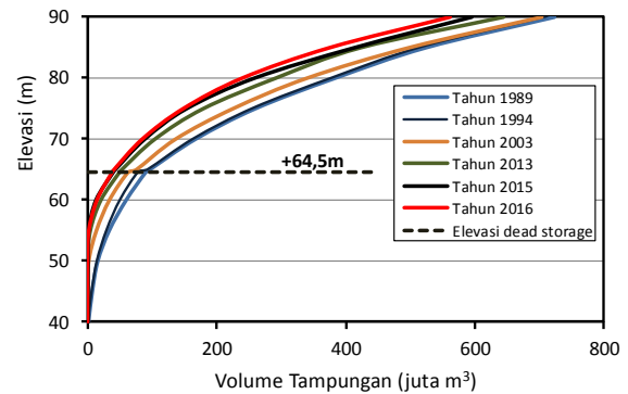
Gambar 8. Kurva karakteristik Waduk Kedungombo
