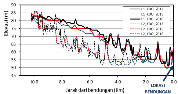
Gambar 14. Perubahan dasar Waduk Kedungombo
