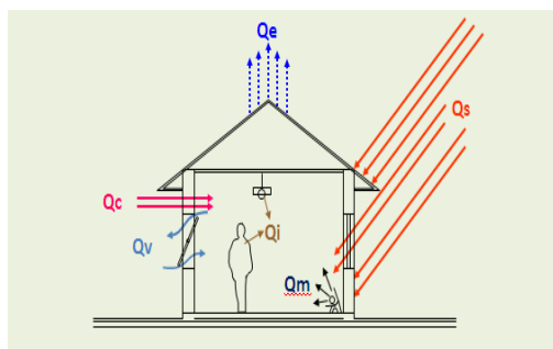
Gambar 06 : pengendalian termal Sumber : Szokolay, 1998
