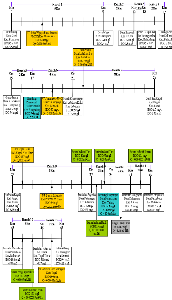
Gambar 1 Skema Pembagian Segmen Sungai Gung dan Lokasi Titik Sampling Sumber : Hasil Analisa, 2007
