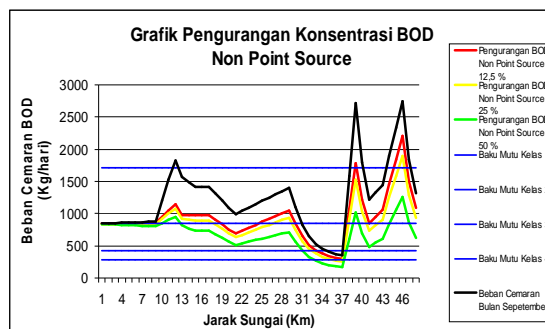
Gambar 14 Hasil Simulasi Pengurangan Cemaran BOD Menu Incremental Inflow
