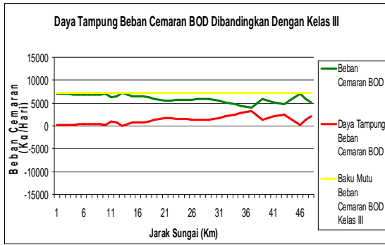
Gambar 11 Daya Tampung Beban Cemaran Sungai Gung Pada Debit Terbesar Bila Dibandingkan Dengan Kelas 3 Sungai
