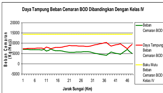
Gambar 12 Daya Tampung Beban Cemaran Sungai Gung Pada Debit Terbesar Bila Dibandingkan Dengan Kelas 4 Sungai
