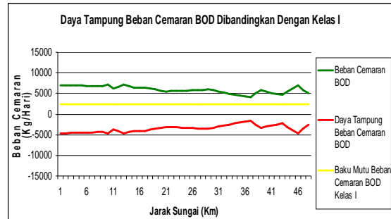
Gambar 9 Daya Tampung Beban Cemaran Sungai Gung Pada Debit Terbesar Bila Dibandingkan Dengan Kelas 1 Sungai
