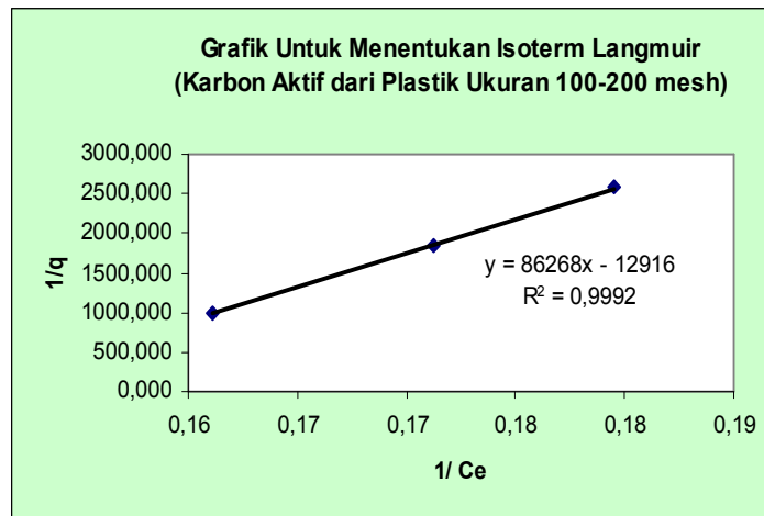
Gambar 7. Penentuan Isoterm Langmuir (Karbon Aktif dari Plastik Ukuran 100-200 mesh)
