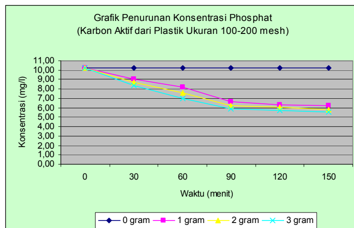
Gambar 1. Penurunan Konsentrasi Phosphat (Karbon Aktif dari Plastik Ukuran 100-200 mesh)
