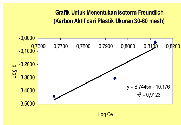
Gambar 6. Penentuan Isotherm Freundlich (Karbon Aktif dari Plastik Ukuran 30-60 mesh)
