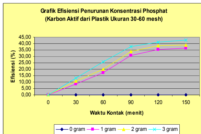
Gambar 4. Efisiensi Penurunan Konsentrasi Fosfat (Karbon Aktif dari Plastik Ukuran 30-60 mesh)
