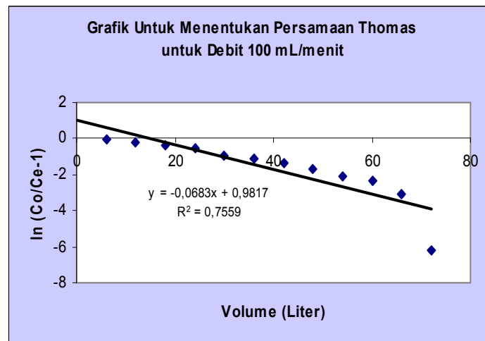
Gambar 14. Penentuan Persamaan Thomas (2)
