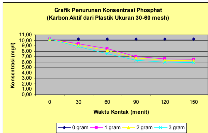
Gambar 3. Penurunan Konsentrasi Fosfat (Karbon Aktif dari Plastik Ukuran 30-60 mesh)
