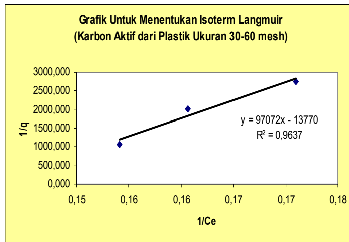
Gambar 8. Penentuan Isoterm Langmuir (Karbon Aktif dari Plastik Ukuran 30-60 mesh)
