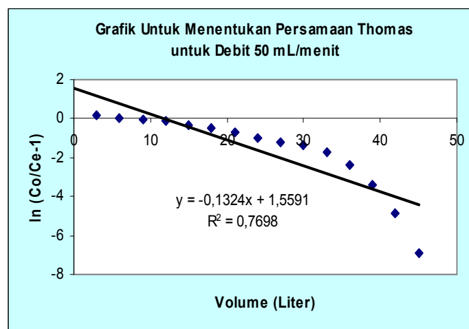
Gambar 13. Penentuan Persamaan Thomas (1)
