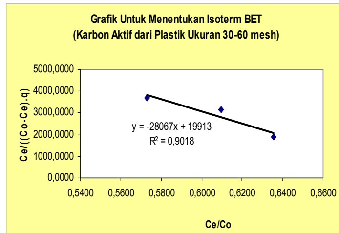
Gambar 10. Penentuan Isoterm BET (Karbon Aktif dari Plastik Ukuran 30-60 mesh)
