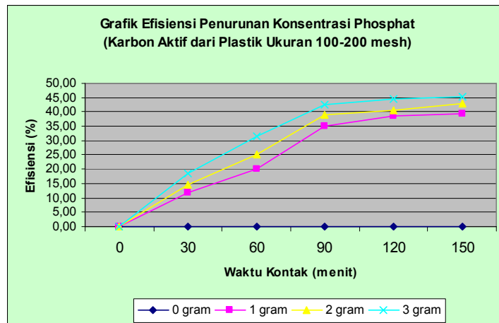
Gambar 2. Efisiensi Penurunan Konsentrasi Fosfat (Karbon Aktif dari Plastik Ukuran 100-200 mesh)
