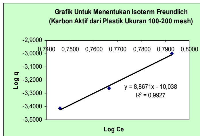
Gambar 5. Penentuan Isotherm Freundlich (Karbon Aktif dari Plastik Ukuran 100-200 mesh)
