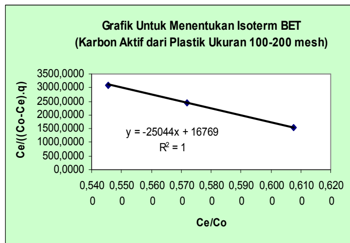
Gambar 9. Penentuan Isoterm BET (Karbon Aktif dari Plastik Ukuran 100-200 mesh)
