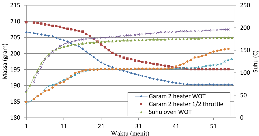
Gambar 5. Grafik Pengujian Gabungan 2 Heater
