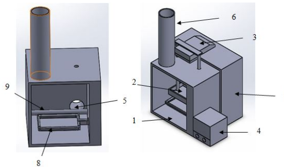
Gambar 2. Skema set up alat
