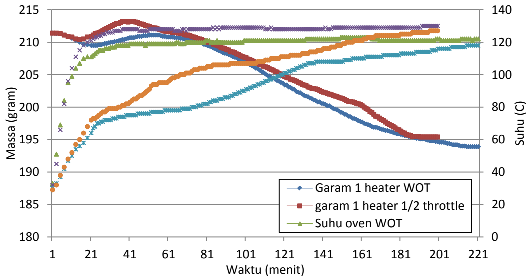
Gambar 4. Grafik Pengujian Gabungan 1 Heater
