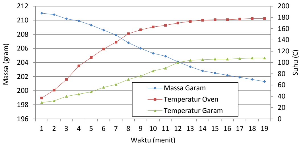
Gambar 6. Pengujian hingga massa garam kembali ke massa awal
