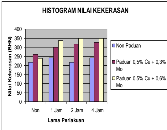
Gambar 3. Histogram Nilai Kekerasan
