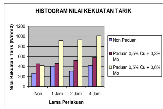
Gambar 2. Histogram Kekuatan Tarik
