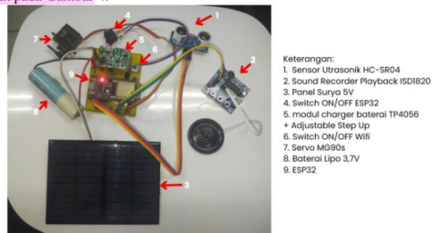
Gambar 4. Hasil perancangan keseluruhan sistem
