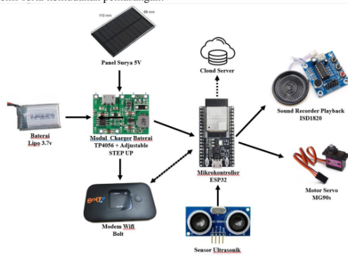
Gambar 2. Wiring diagram perangkat FLOPRO
