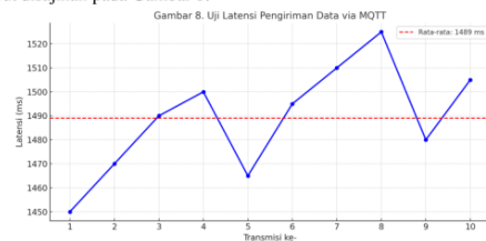
Gambar 8. Uji Latensi Pengiriman Data via MQTT
