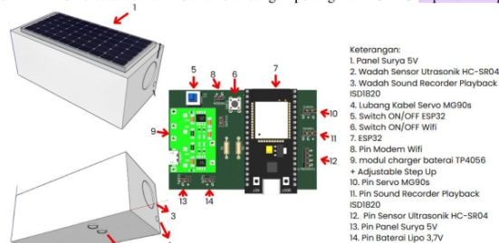
Gambar 1. Rancangan perangkat FLOPRO
