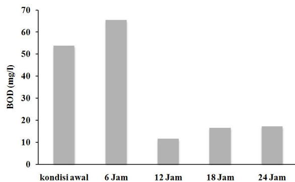
Gambar 3. BOD air kali Banger sebelum dan setelah diproses menggunakan sinar UV + ZnO:KA untuk berbagai lama waktu
