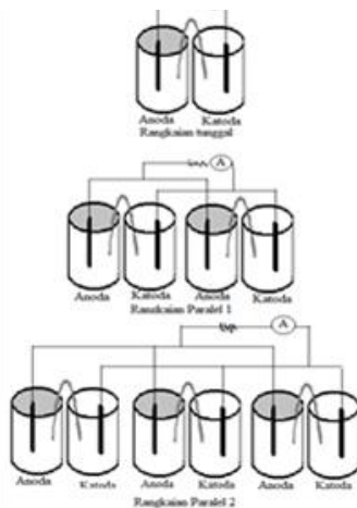
Gambar 1. Skema rangkaian tunggal, paralel 1, dan paralel 2
