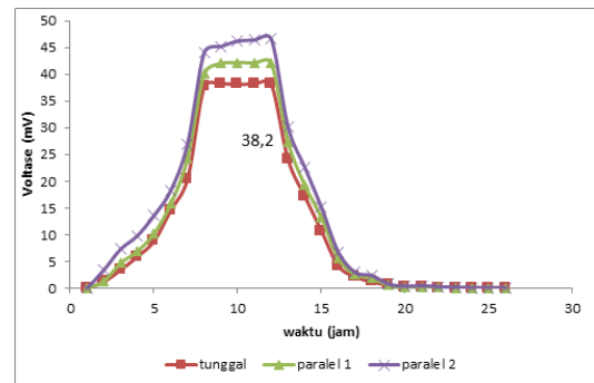
Gambar 4. Beda potensial pada variasi rangkaian paralel dengan substrat Laktosa
