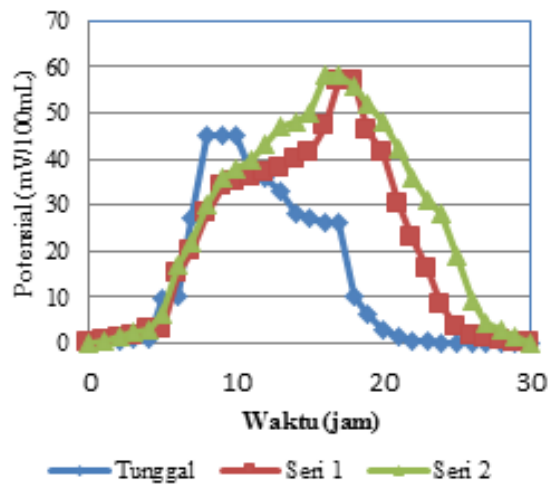
Gambar 1. Beda potensial MFC pada variasi rangkaian seri pada substrat laktosa
