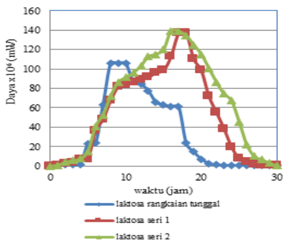
Gambar 2. Daya pada substrat laktosa pada variasi rangkaian seri
