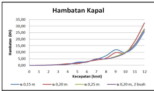
Gambar 7. Grafik hambatan kapal
