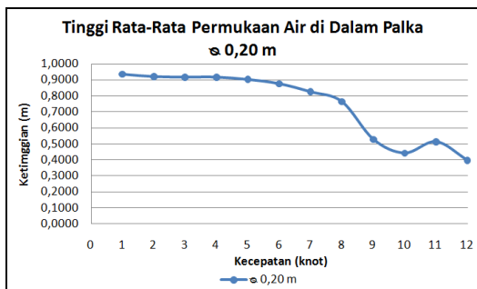
Gambar 15. Tinggi permukaan air di dalam palka sebelum di variasikan (diameter lubang sirkulasi 0,20 m)
