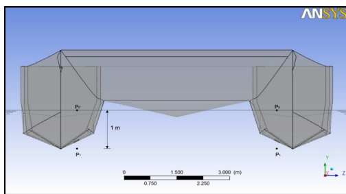
Gambar 10. Letak Posisi Titik Tekanan Tampak Depan
