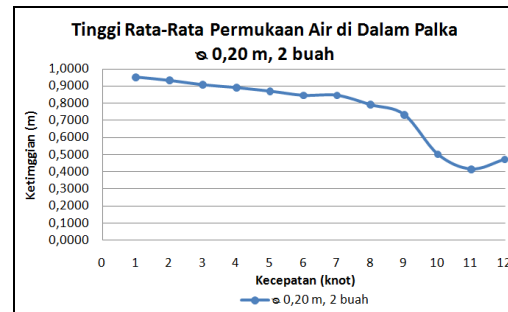
Gambar 17. Tinggi permukaan air di dalam palka sesudah di variasikan (diameter lubang sirkulasi 0,20 m, 2 buah)
