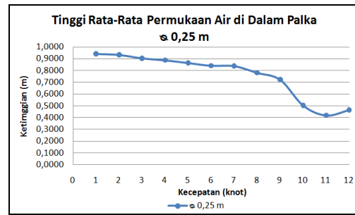
Gambar 17. Tinggi permukaan air di dalam palka sesudah di variasikan (diameter lubang sirkulasi 0,25 m)
