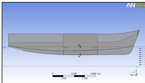
Gambar 8. Letak Posisi Titik Tekanan Tampak Samping
