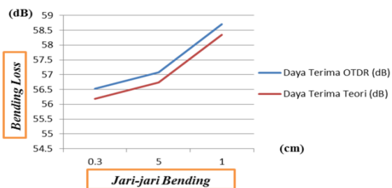
Gambar 13. Grafik Perbandingan Daya Terima Teori Menggunakan PLB Dengan Serat-2
