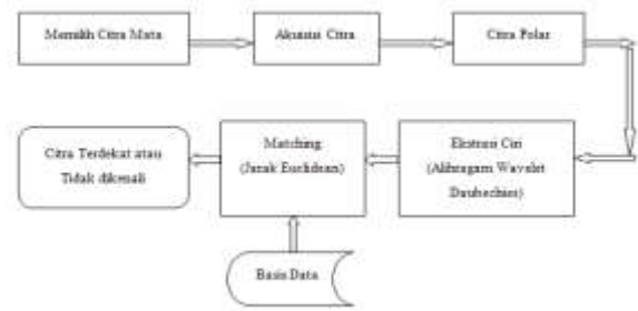
Gambar 3.1 Diagram Alir Sistem Pengenalan Citra Iris Mata menggunakan alihragam wavelet Daubechies orde 4
