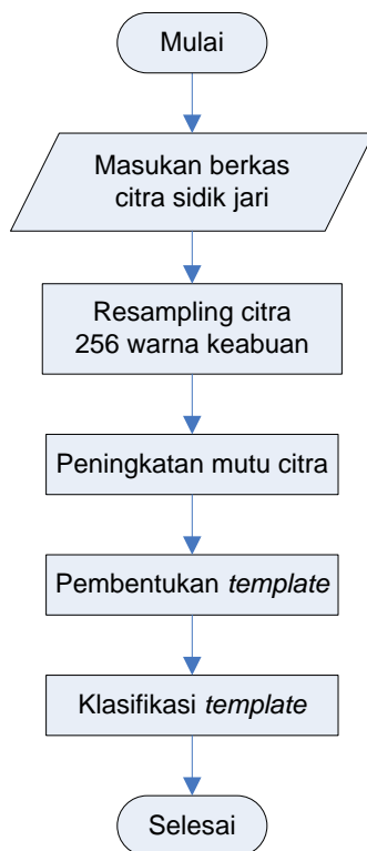
Gambar 3. Diagram alir menu utama
