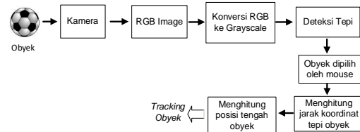
Gambar 2. Blok diagram alur ekstraksi fitur obyek
