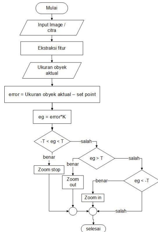
Gambar 7. Flowchart mekanisme zoom
