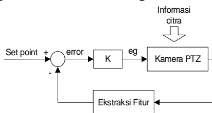
Gambar 6. Blok Diagram Sistem Kontrol Zoom
