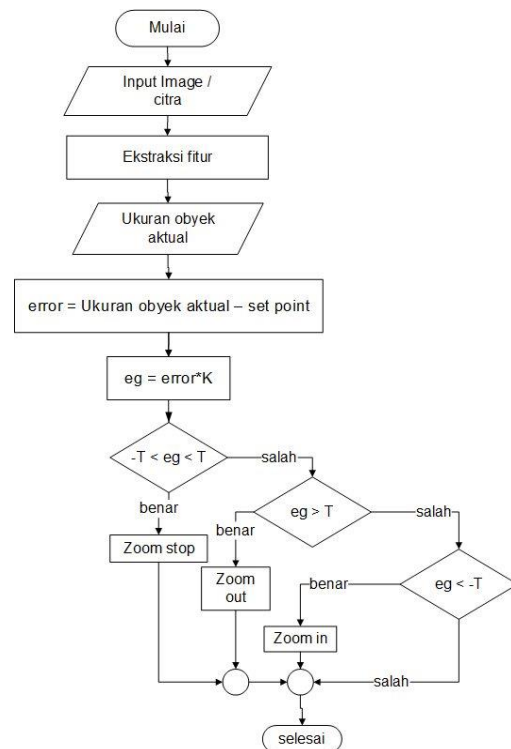
Gambar 7. Flowchart mekanisme zoom
