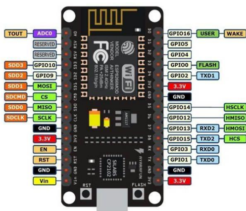
Gambar 1. ESP8266 Node MCU
