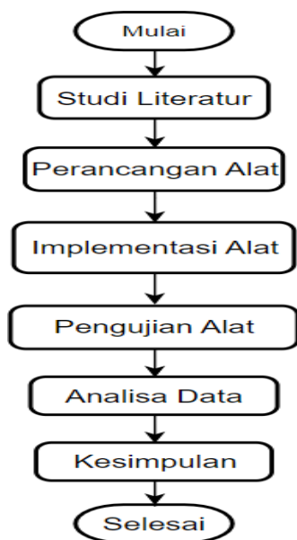
Gambar 7. Tahapan Penelitian
